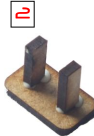
2 Verbindungsstück: Die kleinen Stifte in die abgerundete Platte einkleben. Die breite Seite der Stifte parallel zur kurzen Kante der Platte. Auf rechte Winkel achten.
